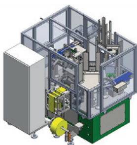
BTR 10 - Macchina confezionatrice. Confeziona il burro in vaschette con coperchio. Prodotto: burro in formato per hotel BTR 10 - Packaging machine. Bundling butter for tray and hood. Product: butter size hotel
