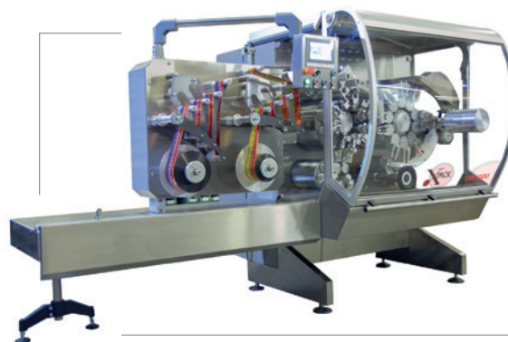
Macchina incartatrice per dadi e cubetti a velocità 1.000. Moto continuo. Cambio formato da dado a cubetto e viceversa Wrapping machine for stock tablet and cubes at speed 1,000. Continuous motion. Size change from tablet to cube, and vice versa
